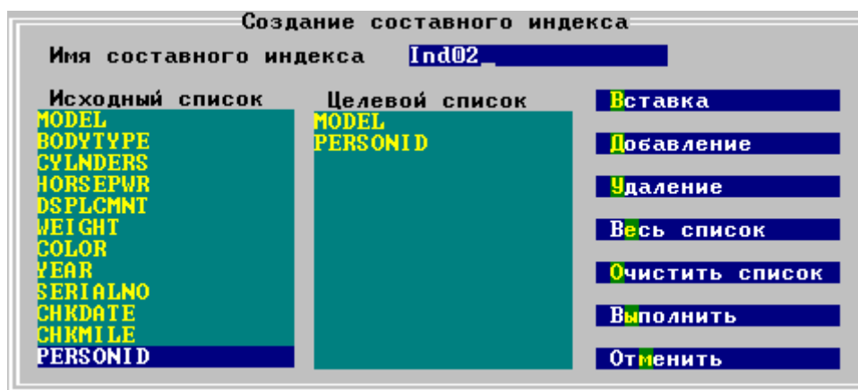
Рис. 32. Окно создания составного индекса
