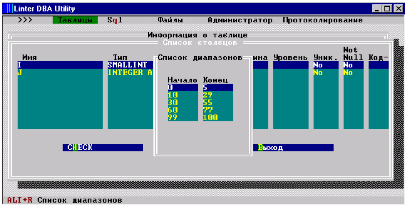
Рис. 9. Список диапазонов для AUTOINC
