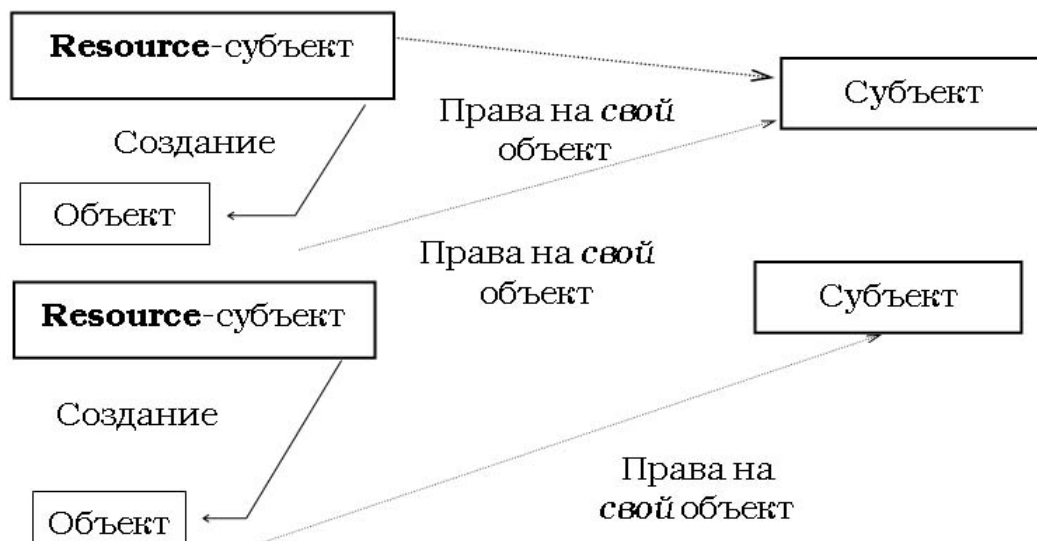
Рис. 1. Схема прямой передачи доступа в СУБД ЛИНТЕР
