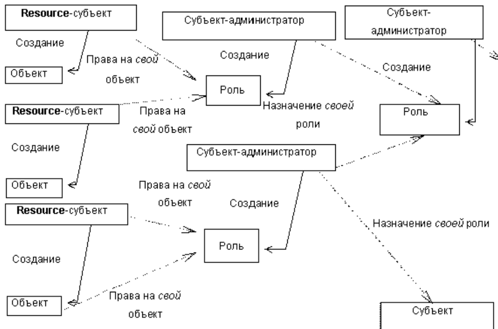
Рис. 2. Схема построения ролей в СУБД ЛИНТЕР
