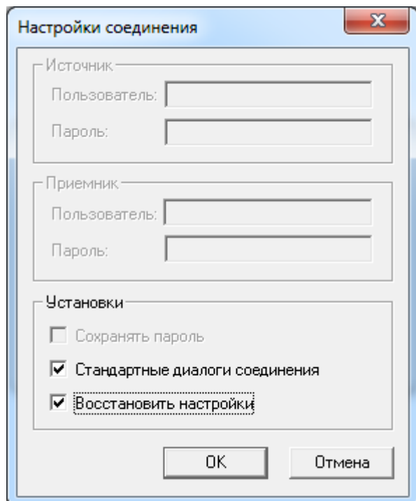
Рисунок 2. Настройки соединения
