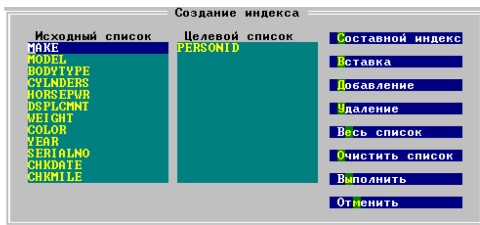
Рисунок 29. Создание индекса
