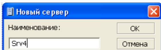
Рисунок 5. Создание сервера
