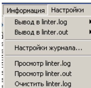
Рисунок 9. Управление протоколированием
